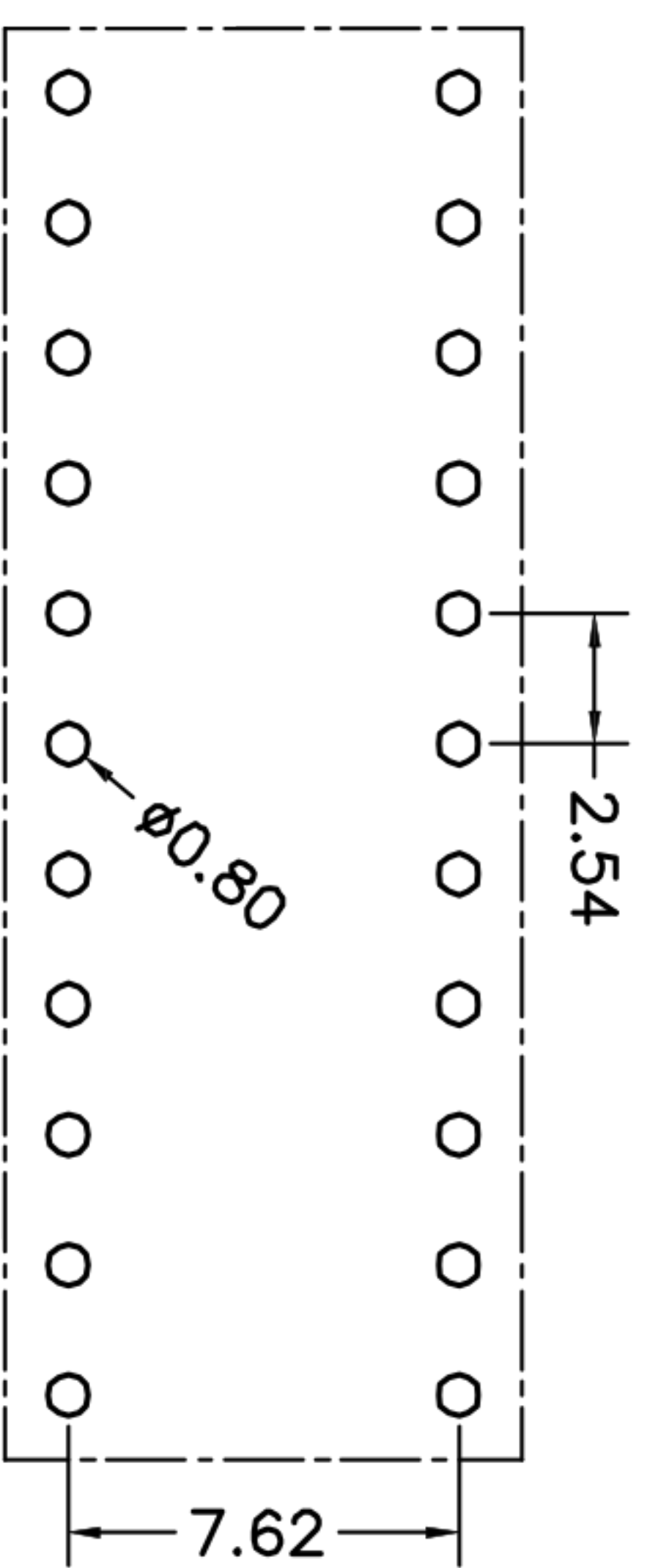
P.C.B LAYOUT
